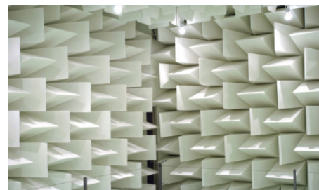
▲ Salle semi-anechoïque « Marin Mersenne » (SSA) : enceinte isolée dont les murs et le plafond sont capitonnés pour absorber l'énergie acoustique incidente.
