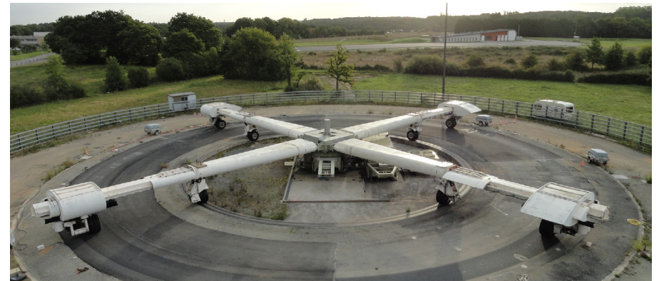
▲ The Pavement Fatigue Carousel.
